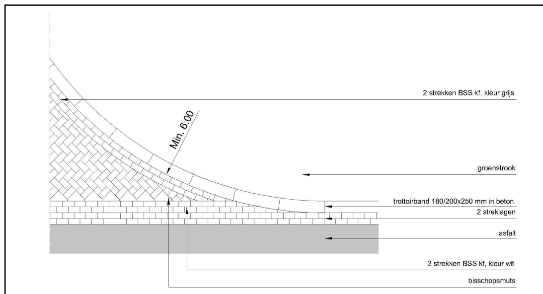
Standaard inritconstructie t.b.v. bedrijfsmatig gebruik type 2
