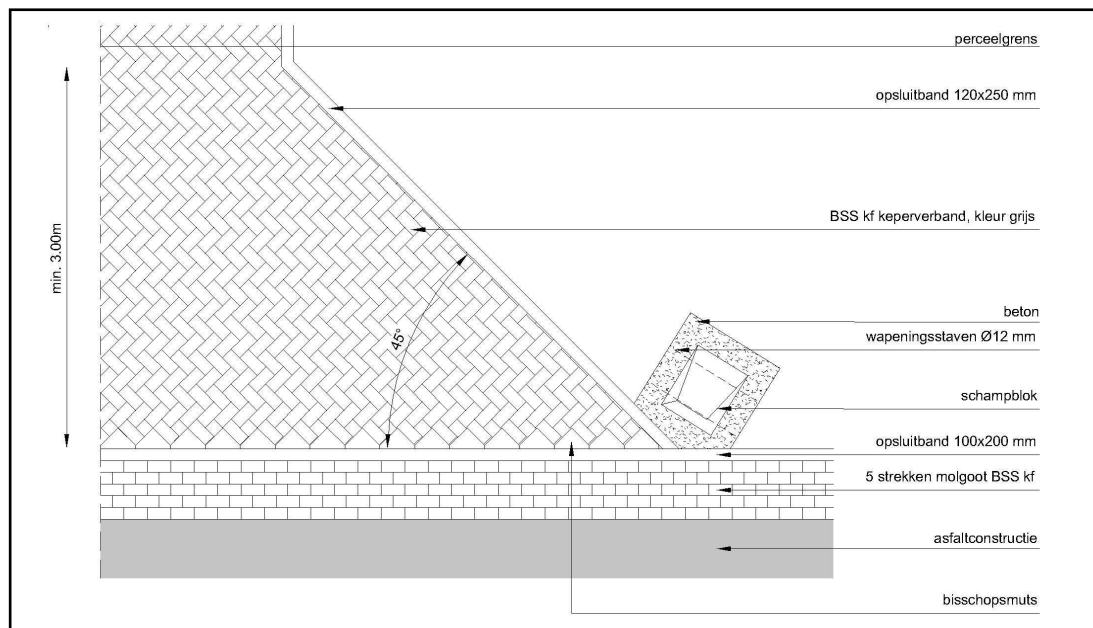
Standaard inritconstructie t.b.v. bedrijfsmatig gebruik type 1
