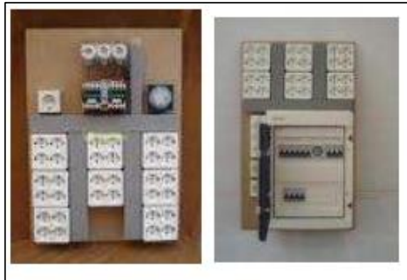
Figuur 4. Schakelborden
