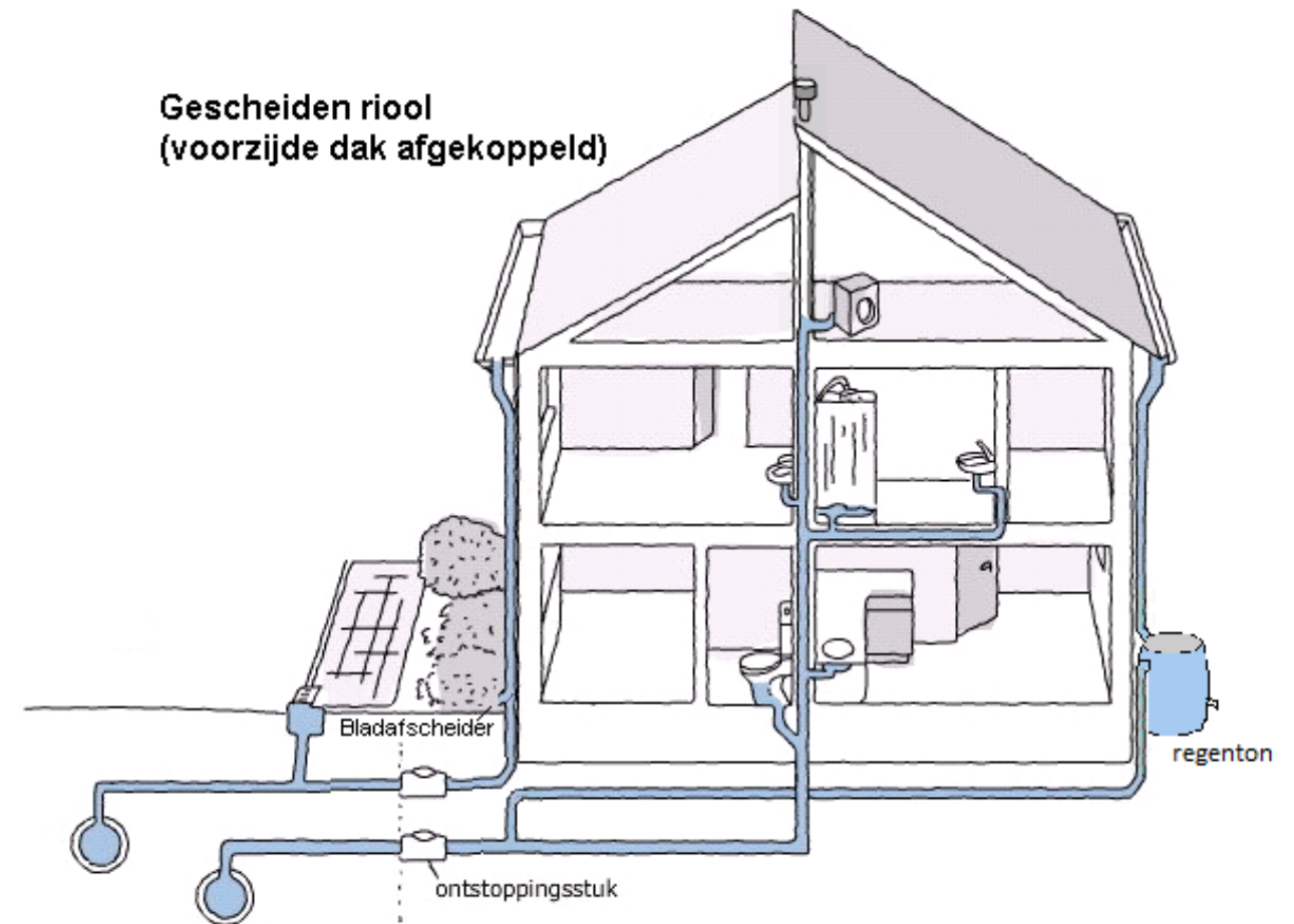
Afkoppelen regenwater
