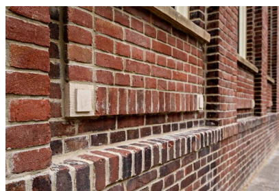
Duidelijke hiërarchie en plasticiteit in de gevel, door diepe negges en (baksteen)verspringing.
