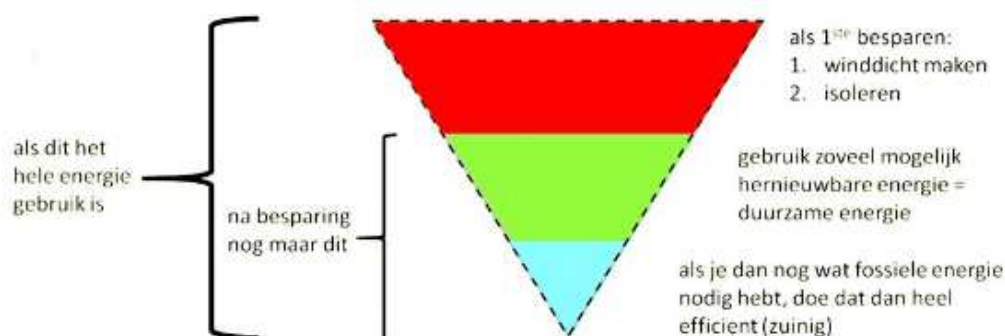
Figuur 24: Trias energetica 42
