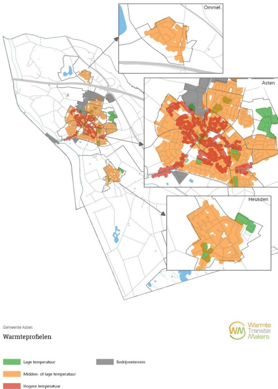
Figuur E: Warmteprofielen gemeente Asten: de afgifte-temperatuur die nodig is nadat alle rendabele isolatiestappen gezet zijn. We geven clusters weer van huizen met eenzelfde warmteprofiel. Individuele huizen zijn niet in kaart gebracht.
