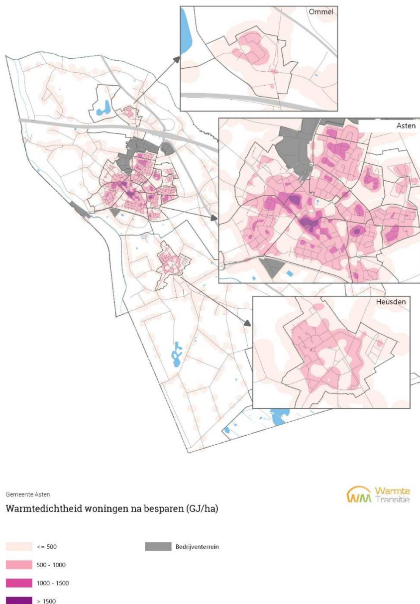
Figuur 14: De verwachte toekomstige warmtedichtheid in gemeente Asten. De warmtedichtheid is gebaseerd op de warmtevraag die over blijft na besparingsmaatregelen.
