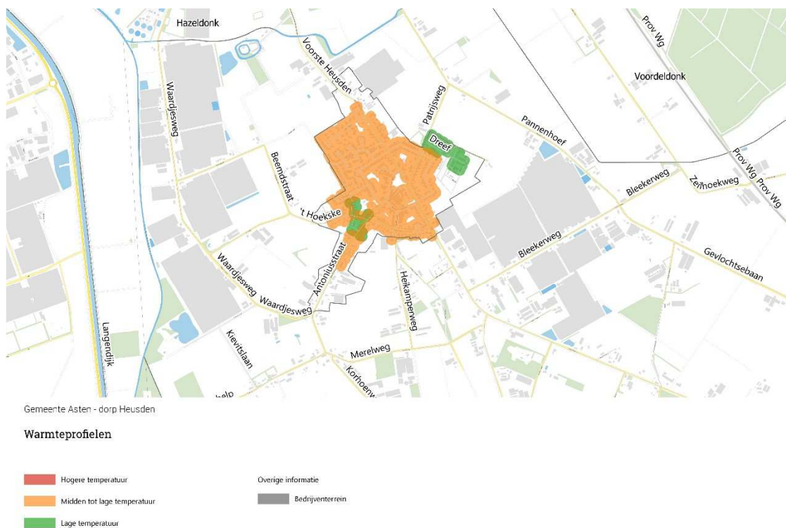
Figuur 12 warmteprofiel kern Heusden
