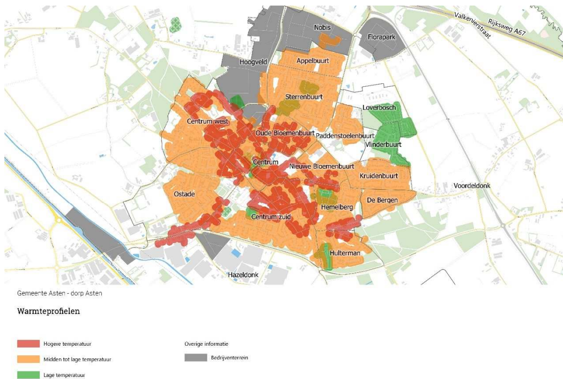
Figuur 11 warmteprofiel kern Asten
